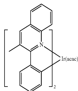
Ir(3-Mepq) 2 (acac)
