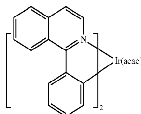
Ir(piq) 2 (acac)
